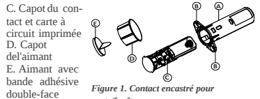
Figure 1. Contact encastré pour porte/fenêtre
