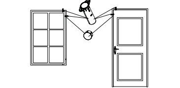
Figura 5. Marque la ubicación del contacto para ventana/puerta y del imán. Asegúrese de que las ubicaciones del contacto y del imán estén alineadas correctamente.
