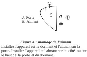
Figure 4 : montage de l'aimant Installez l'appareil sur le dormant et l'aimant sur la porte. Installez l'appareil et l'aimant sur le côté ou sur le haut de la porte et du dormant.
