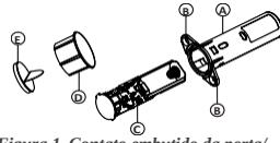
Figura 1. Contato embutido da porta/-janela
