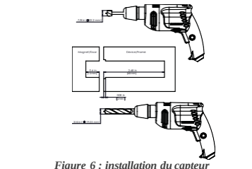
Figure 6 : installation du capteur
